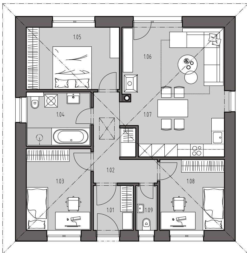
PÔDORYS 1NP
