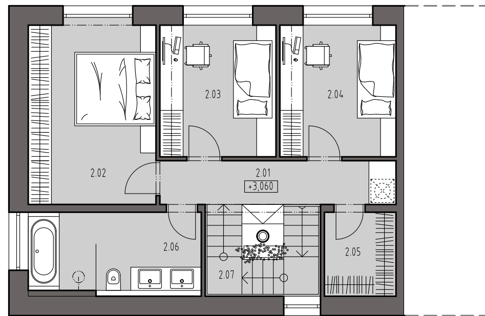
PÔDORYS 2NP
