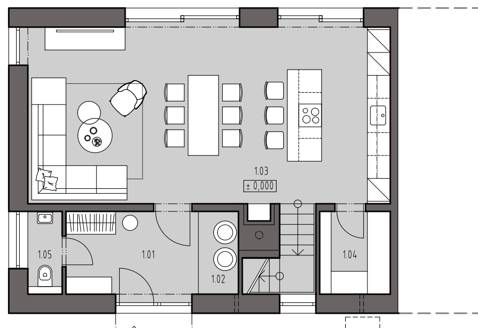
PÔDORYS 1NP
